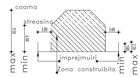
PROFIL LONGITUDINAL L-L
