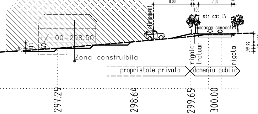
PROFIL LONGITUDINAL L-L
